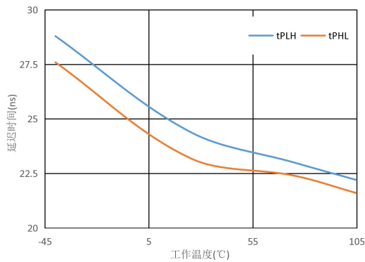
图7.驱动器延时 vs. 工作温度
