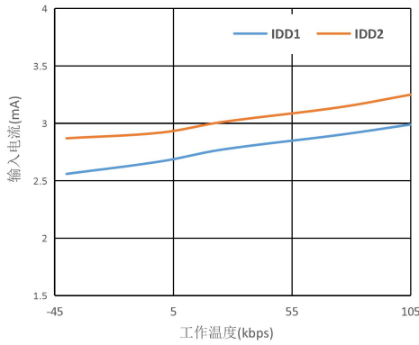
图3. 空载输入电流 vs. 工作温度
