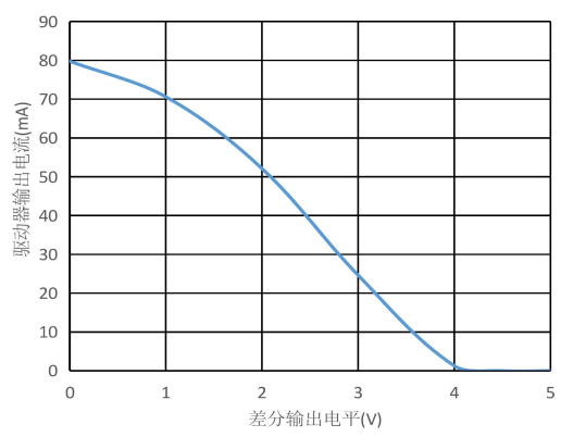
图6. 驱动器输出电流 vs. 差分输出电平
