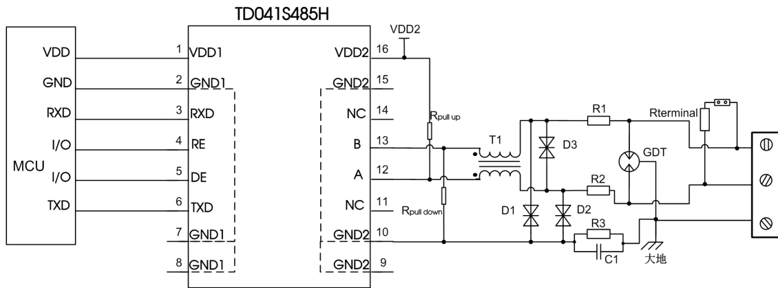
图 14 端口保护推荐电路
