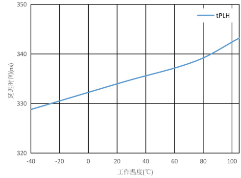
图4. 驱动器延时 vs. 工作温度
