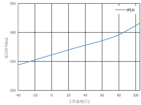
图4. 驱动器延时 vs. 工作温度
