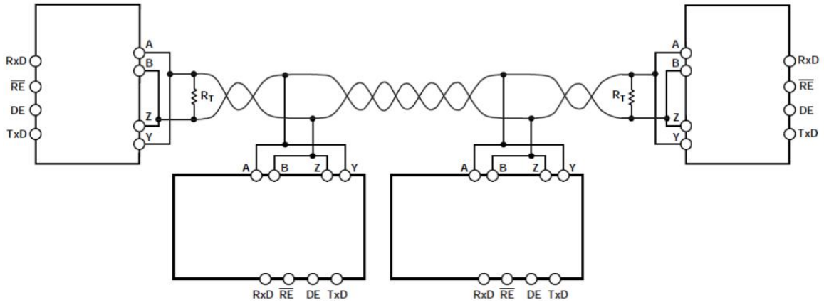
图 10.典型应用电路（半双工网络拓扑结构）
