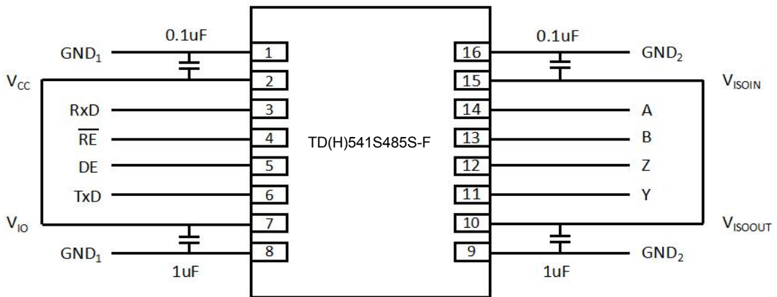
图 12.典型应用PCB layout
