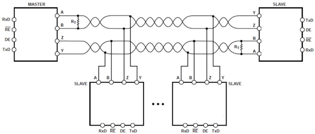
图 11.典型应用电路（全双工网络拓扑结构）
