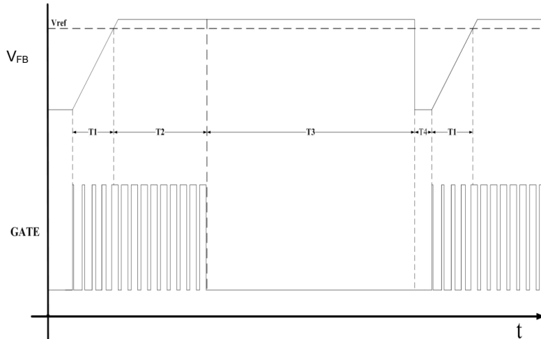
图 17 输出短路时 V_{FB} 与 GATE 的时序图
