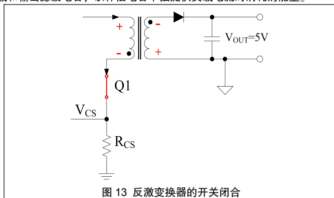
图 13 反激变换器的开关闭合
