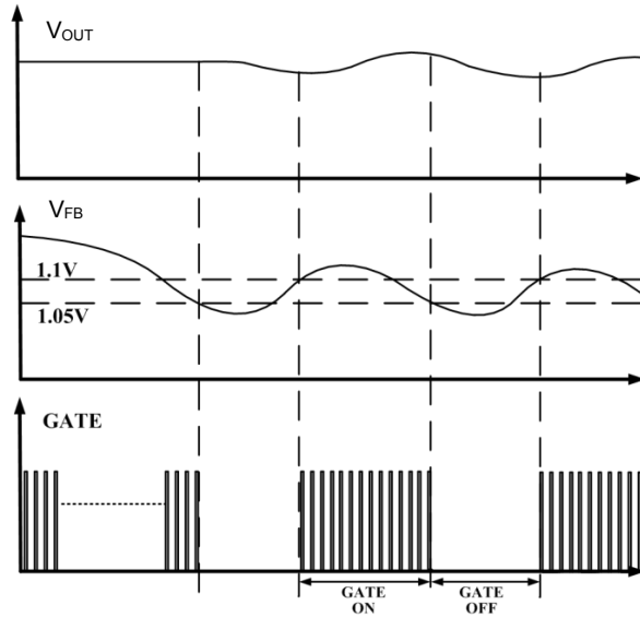
图 16 间歇工作模式时序图
