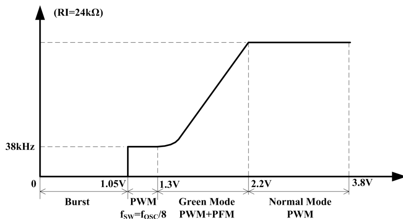
图 15 FB 引脚电压与输出频率的关系
