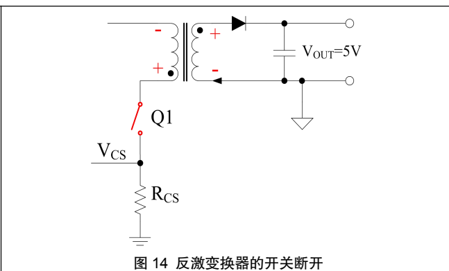
图 14 反激变换器的开关断开
