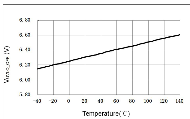
图 2 欠压锁定开启 VS 温度
