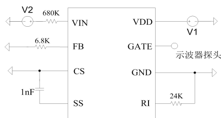
图 12 电学特性测试电路原理图
