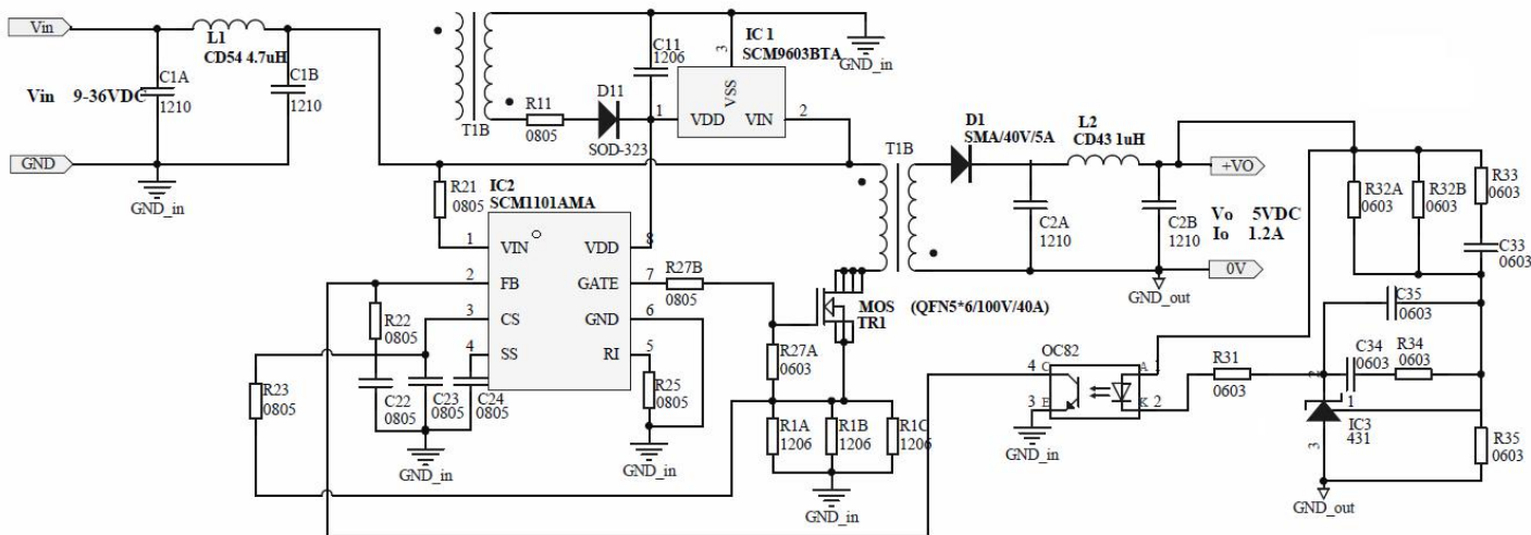
图 19 应用电路
