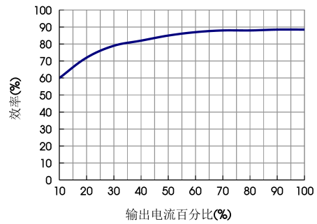
效率Vs输出负载 (Vin=15V)
