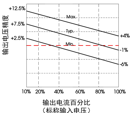
QA053C-2004R3S 主路误差包络曲线图
