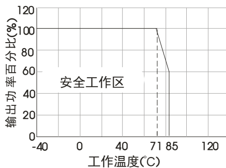
温度降额曲线
