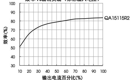
效率 Vs 输出负载 (标称输入电压)
