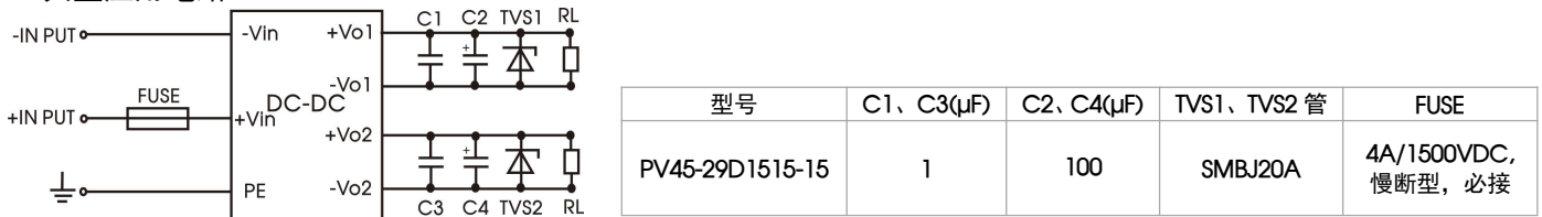
图 1: 典型应用电路
