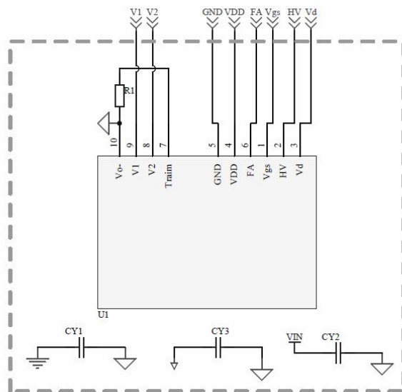
LSC15-26Dxx 核心板
