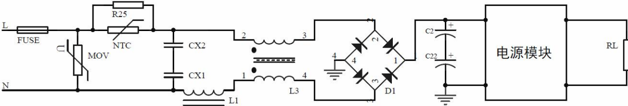
推荐电路 4
