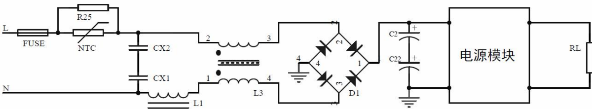
推荐电路 2
