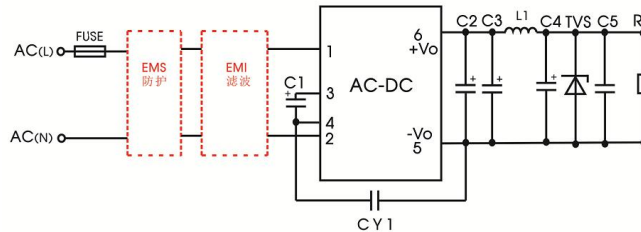
LS 系列外围总体方案设计
