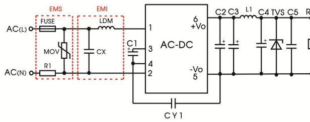
应用电路 4
