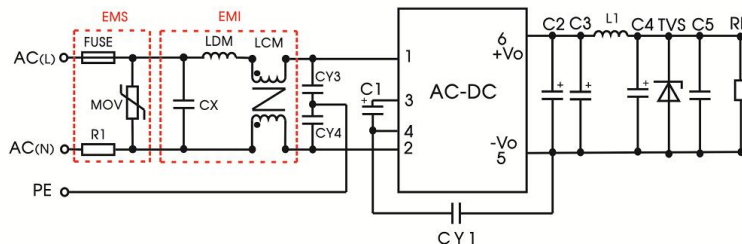
应用电路 5
