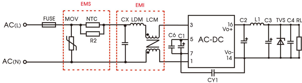
推荐电路 3
