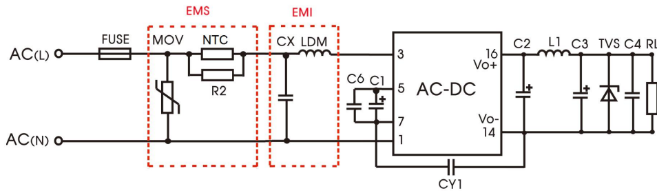
推荐电路 4
