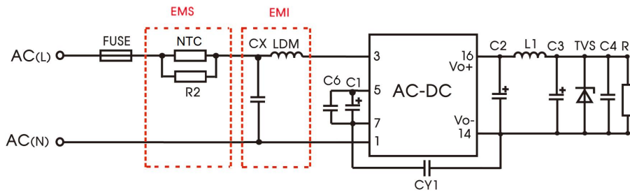
推荐电路 1
