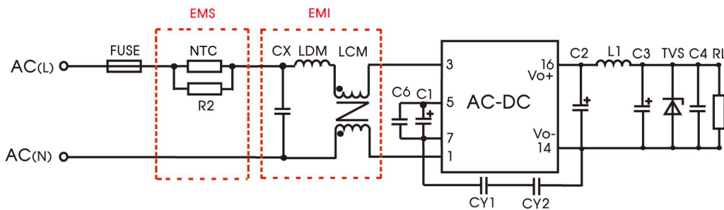
推荐电路 2
