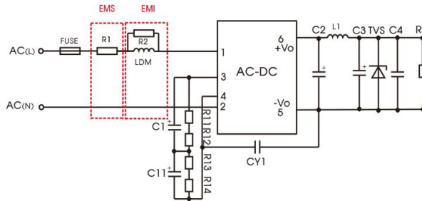
推荐电路 1
