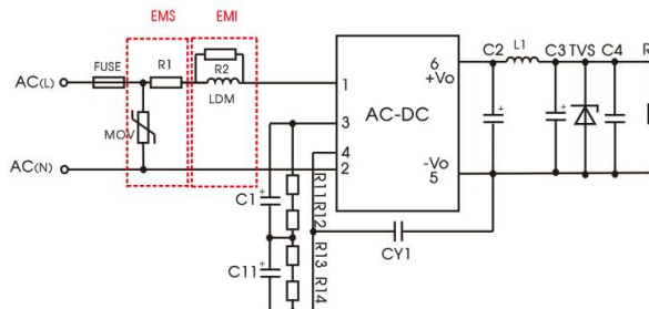
推荐电路 4
