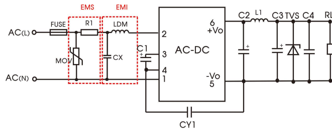
推荐电路 3
