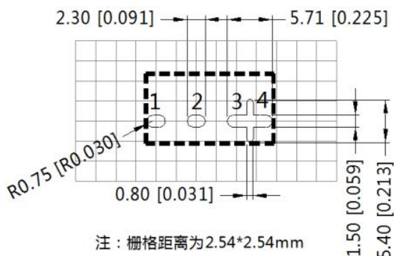
引脚方式
