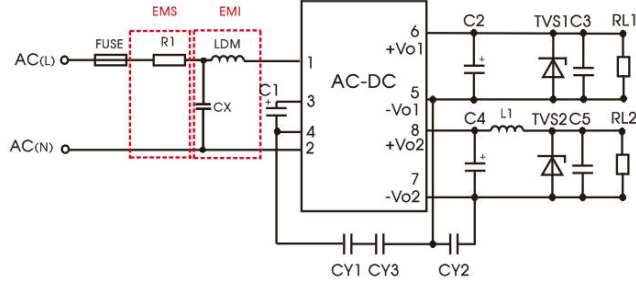
推荐电路 2
