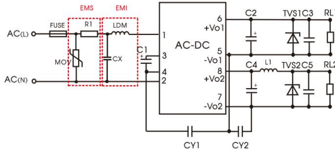
推荐电路 3
