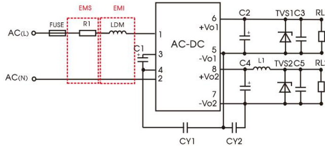
推荐电路 1
