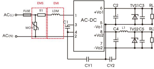
推荐电路 4
