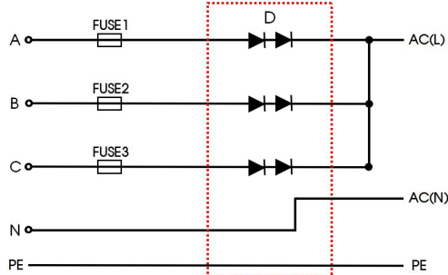
图 3: 推荐电路-半波整流
