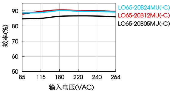
效率Vs输入电压（满载）
