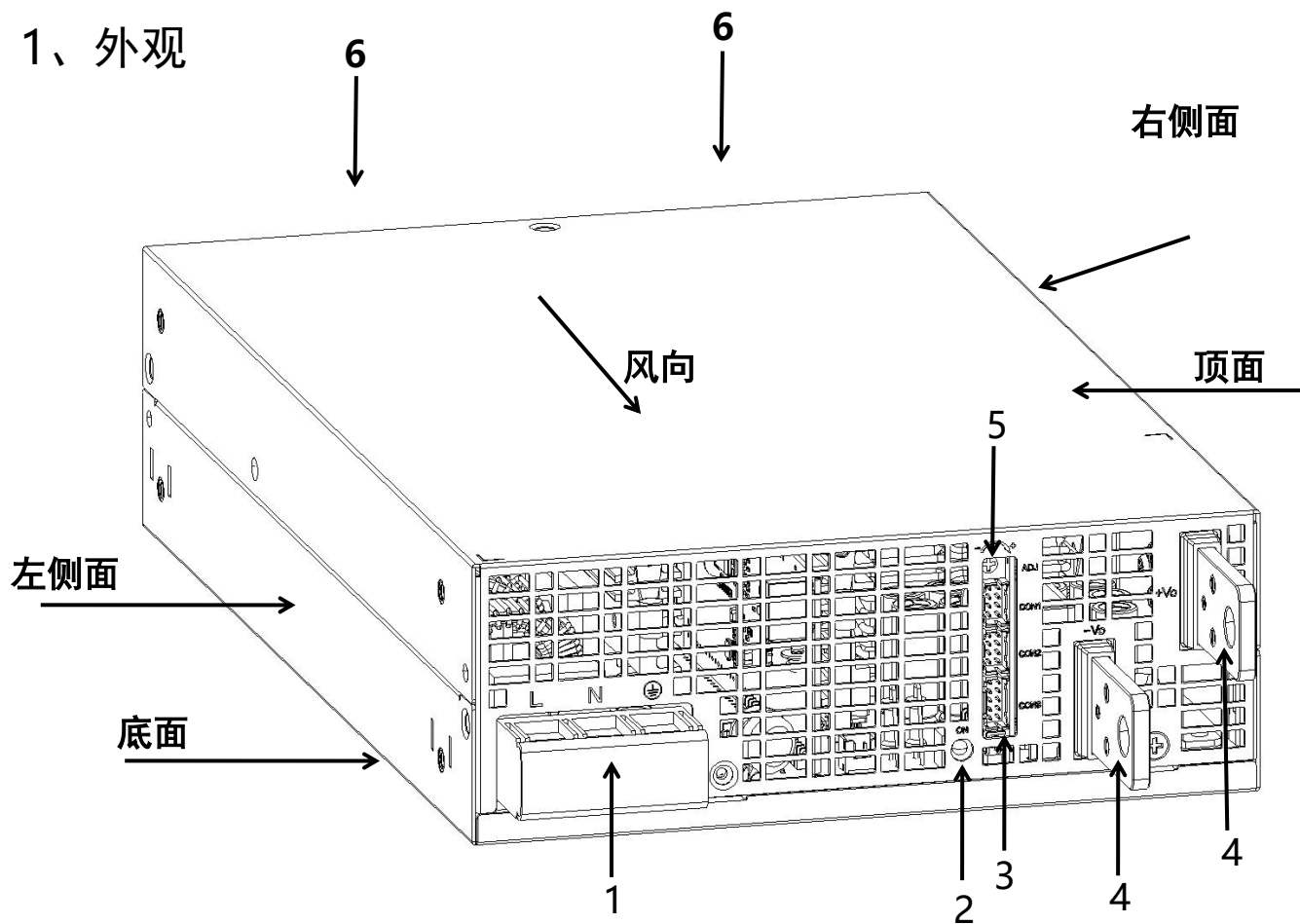
图 1：LMF3000-22Bxx 外观信息
