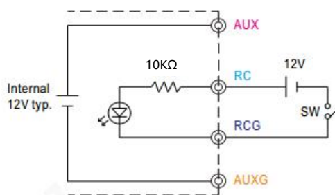
图 1 用外部电压
