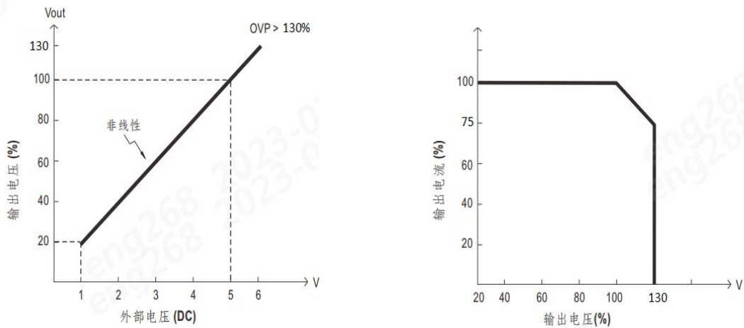
图 2 额定电流随输出电压调整变化
