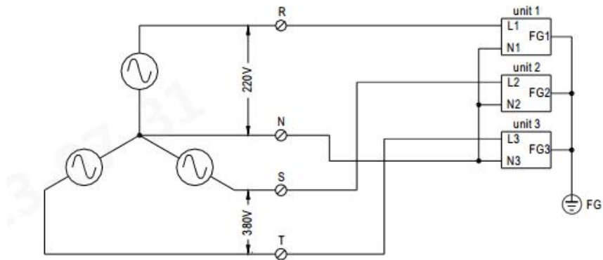
图 2 三相四线 220/380VAC 系统
