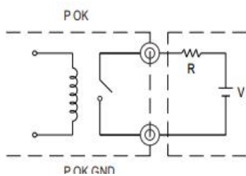
图 1 电源正常的内部回路（继电器，共 10W） （最大吸入电流 500mA，最大电压 20V）
