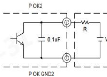
图 2 电源正常的内部回路（集电极开路的方法） （最大吸入电流 10mA，最大电压 30V）
