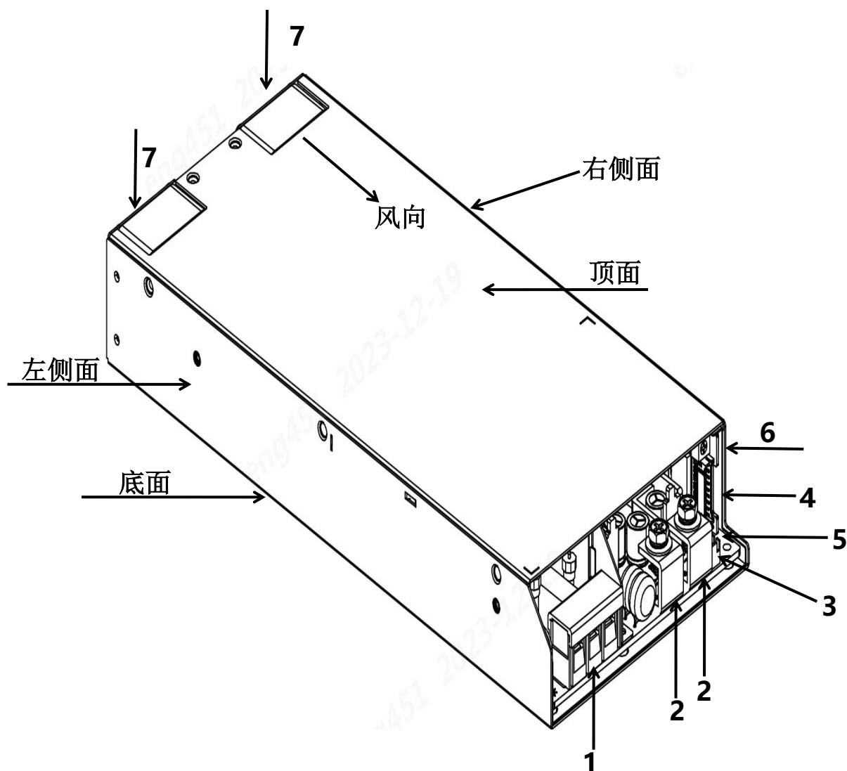
图 1：LMF2000-20Bxx 外观信息
