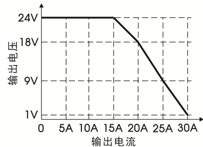
输出电压 VS 输出电流示意图(Typ.)
