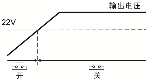
DC OK 动作示意图(Typ.)
