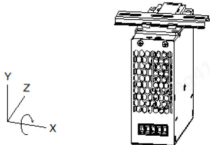
旋转安装位置(270° X-轴)
