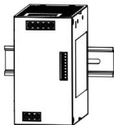
① 端子接上连接线后, 铺设和对齐 连接线; ② 通过外壳两侧的缺口, 用电线捆 扎条, 固定连接线。
