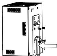
① 安装通用DIN导轨适配器 (侧面正装, 需撕标签纸)
