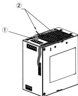
① 端子接上连接线后, 铺设和对齐 连接线; ② 通过外壳两侧的缺口, 用电线捆 扎条, 固定连接线。
