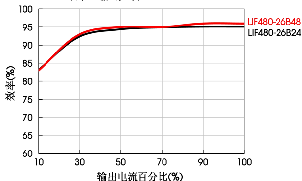
效率Vs输出负载 (Vin=400VAC)
