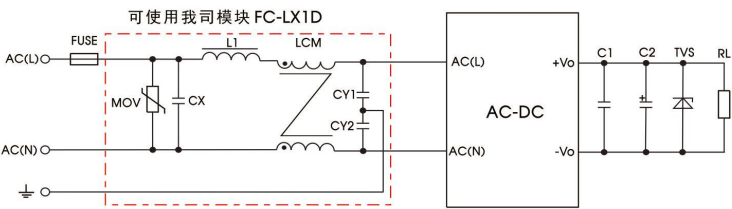
图 2：EMC 更高要求推荐电路
