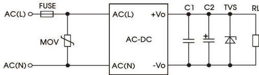
图 1: 典型电路图
