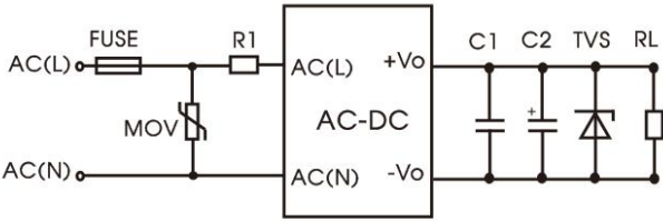
图 2：EMC 更高要求推荐电路
