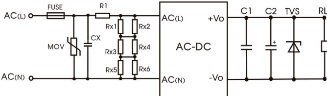
图 2：EMC 更高要求推荐电路
