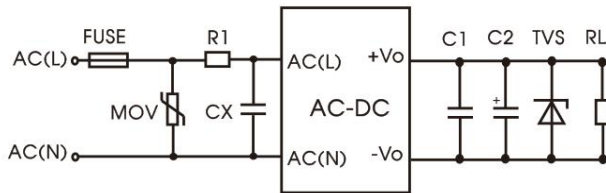
图 2：EMC 更高要求推荐电路
