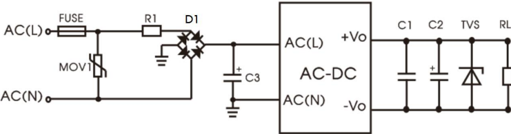
图 3：EMC 更高要求推荐电路
