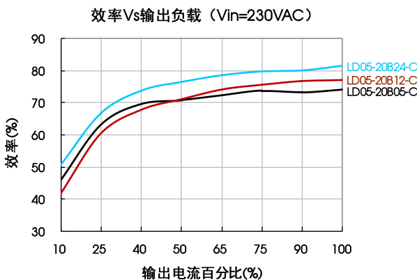
效率Vs输出负载（Vin=230VAC）
