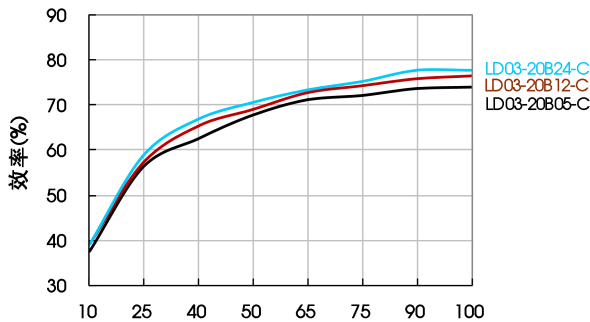
效率Vs输出负载（Vin=230VAC）
