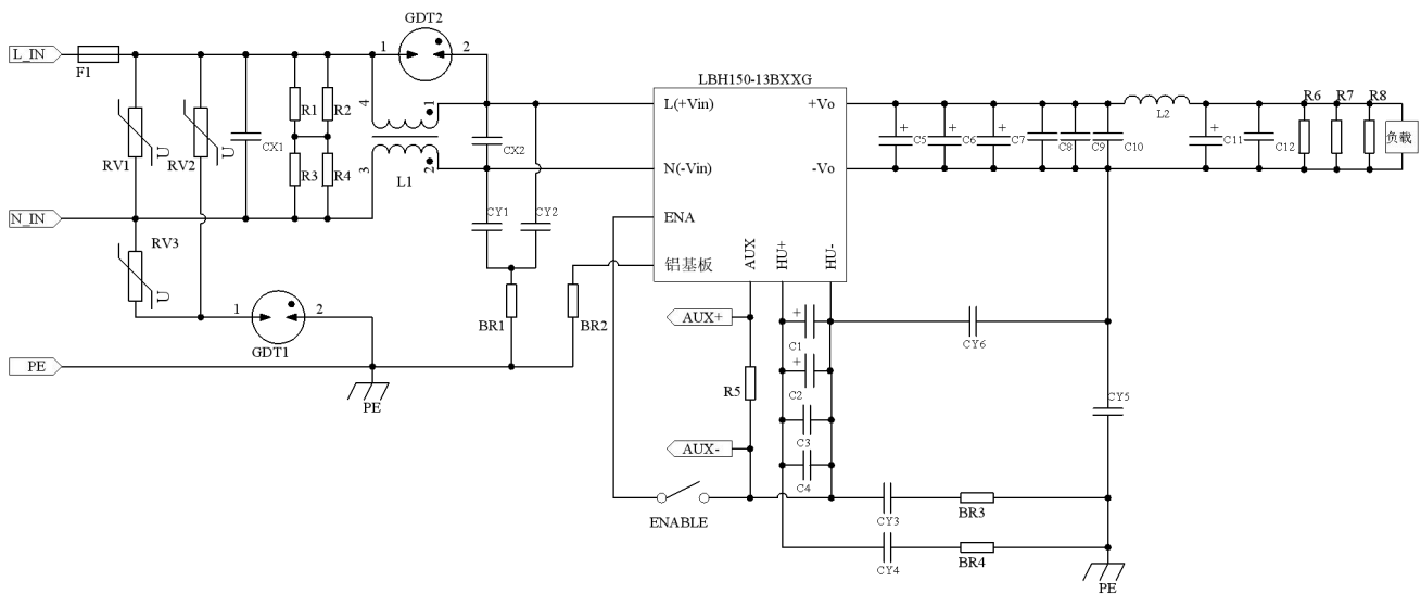
图 1: 推荐电路 1
