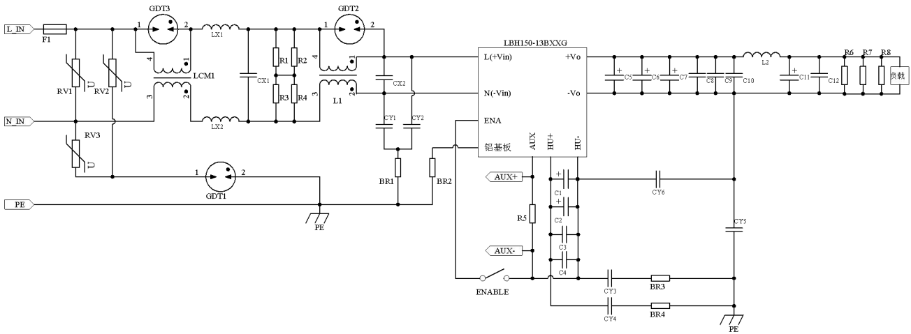
图 2：推荐电路 2
