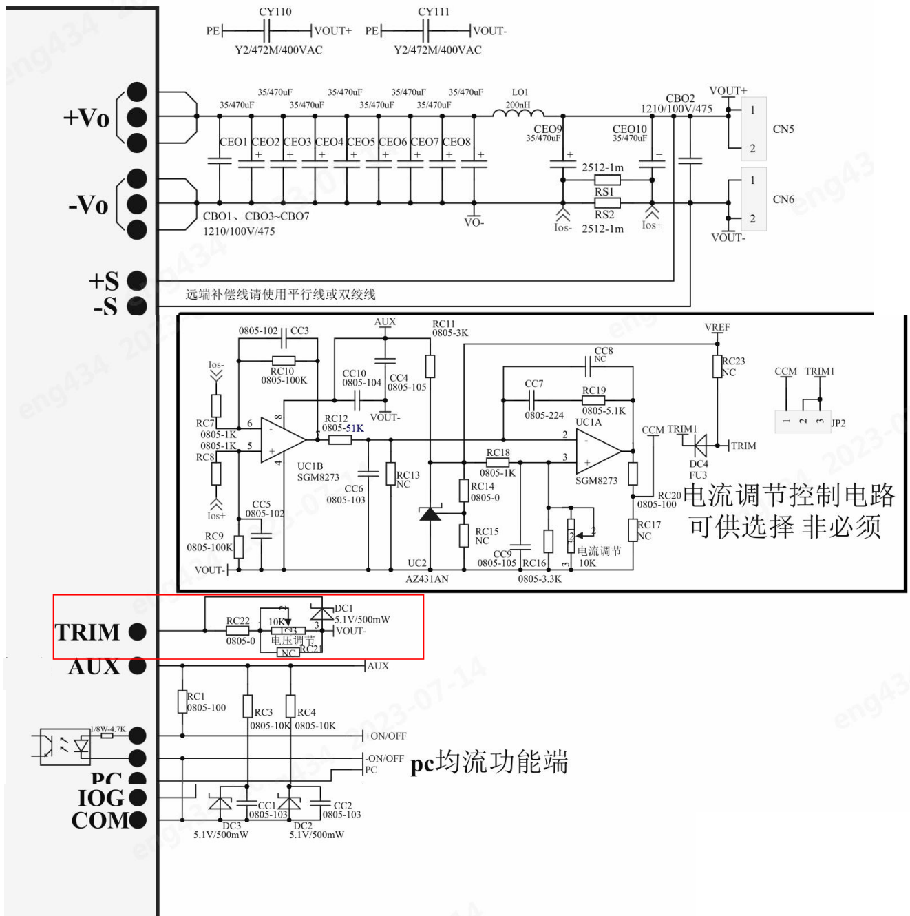
图 3: 输出电压调节连接示意图
