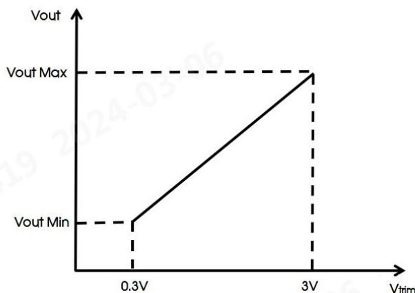
图 4: Vtrim 与 Vout 对应参考曲线图
