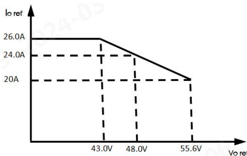
图 9：输出电压给定值与恒流点之间关系图
