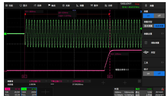
Vin=230VAC 满载启机（启机延迟 634ms）
