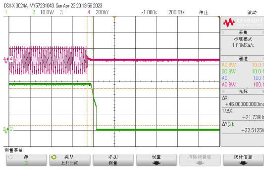
Vin=115VAC 满载关机（掉电保持 46ms）
