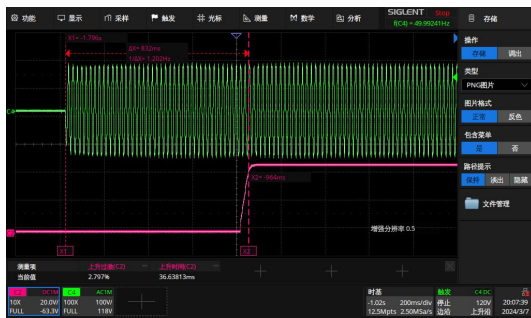
Vin=115VAC 满载启机（启机延迟 832ms）
