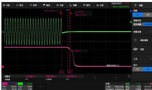
Vin=115VAC 满载关机（掉电保持 65ms）
