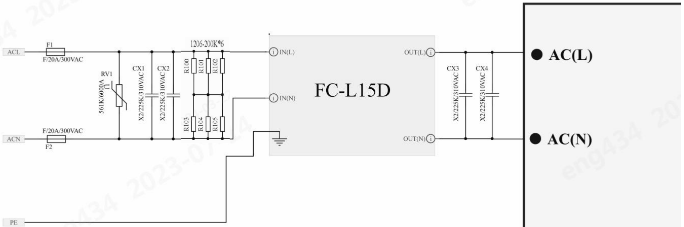
推荐外围电路 3 (EMC 部分)
