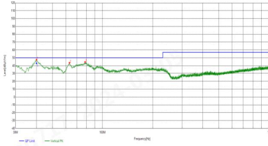
垂直波形及读数
