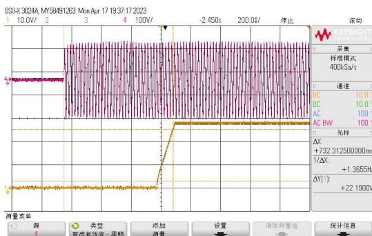
Vin=115VAC 满载启机（启机延迟 732ms）
