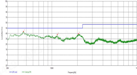
垂直波形及读数
