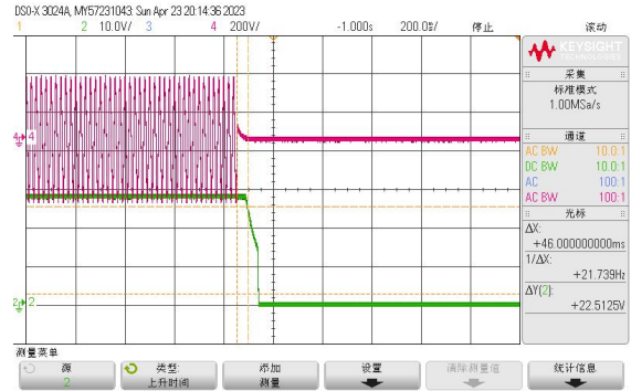
Vin=230VAC 满载关机（掉电保持 46ms）
