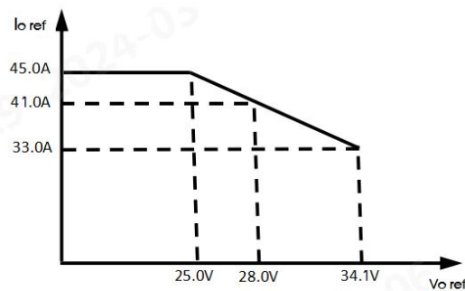
图 8：输出电压给定值与恒流点之间关系图
