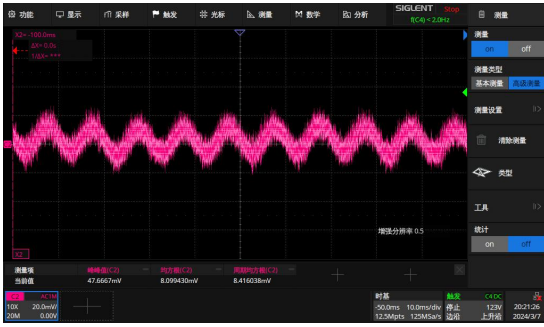
Vin=115VAC 满载纹波噪声(48mV)/纹波有效值(8.1mV)
