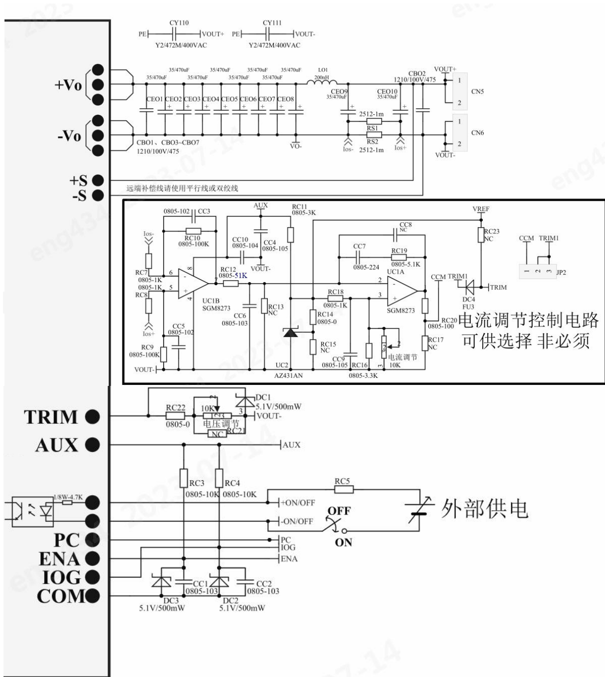
图 7：遥控开关连接示意图
