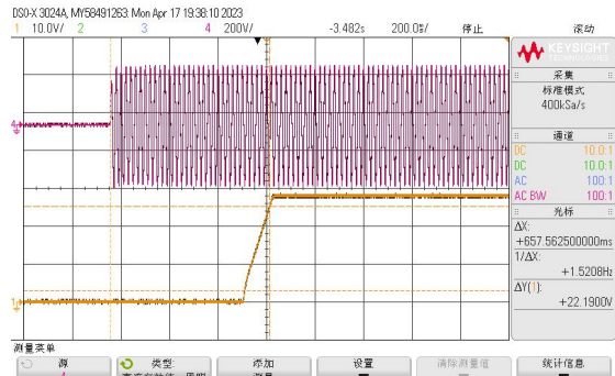
Vin=230VAC 满载启机（启机延迟 657ms）
