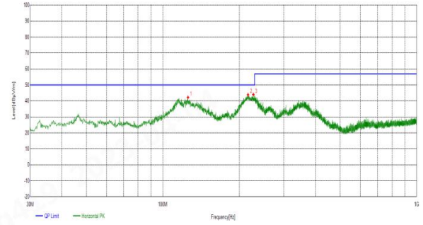
水平波形及读数
