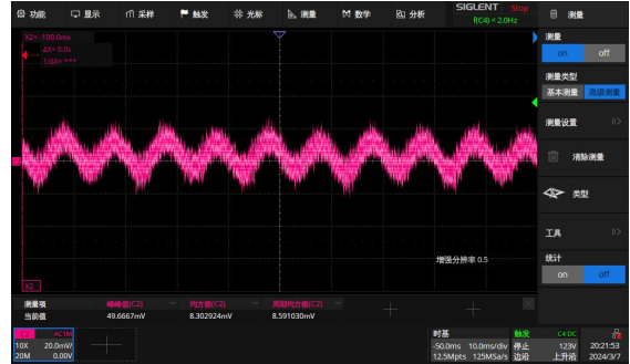
Vin=230VAC 满载纹波噪声(50mV)/纹波有效值(8.6mV)
