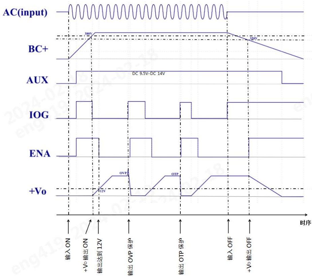
电路时序图
