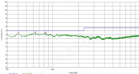
垂直波形及读数
