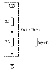
图6 模块内部 Vset 连接图（虚线框）
