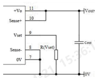
图5 Vset 外接调整电阻接线图
