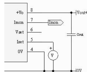
图 8 Iset 外部电源驱动接线图
