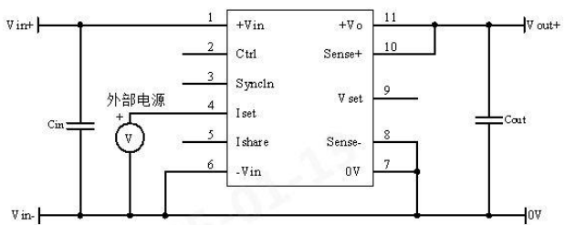
图 8 Iset 外部电源驱动接线图
