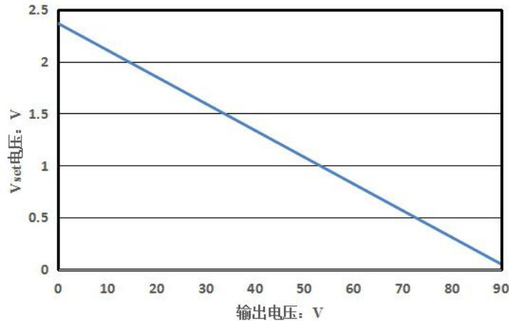
图 3 Vset 电压 VS 输出电压
