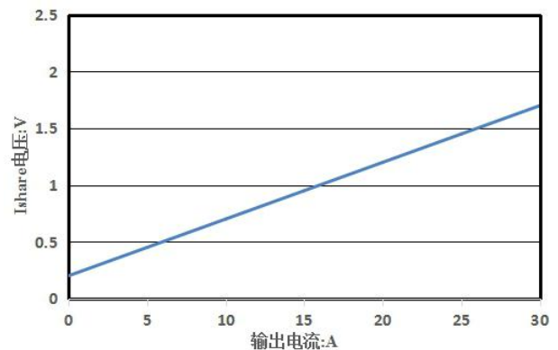
图 10 Ishare VS 输出电流
