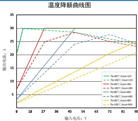
注：控制金属外壳 A 点温度为 80°C 和 100°C 时，最大输出功率降额曲线跟输入电压关系
