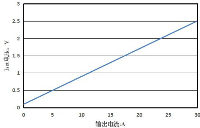
图 7 Iset 电压 Vs 输出电流
