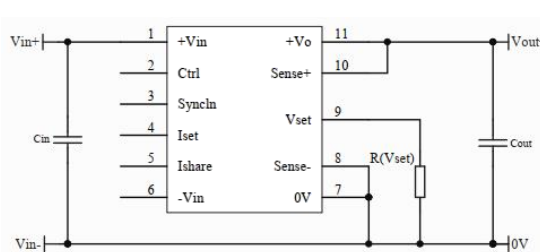
图 5 Vset 外接调整电阻接线图
