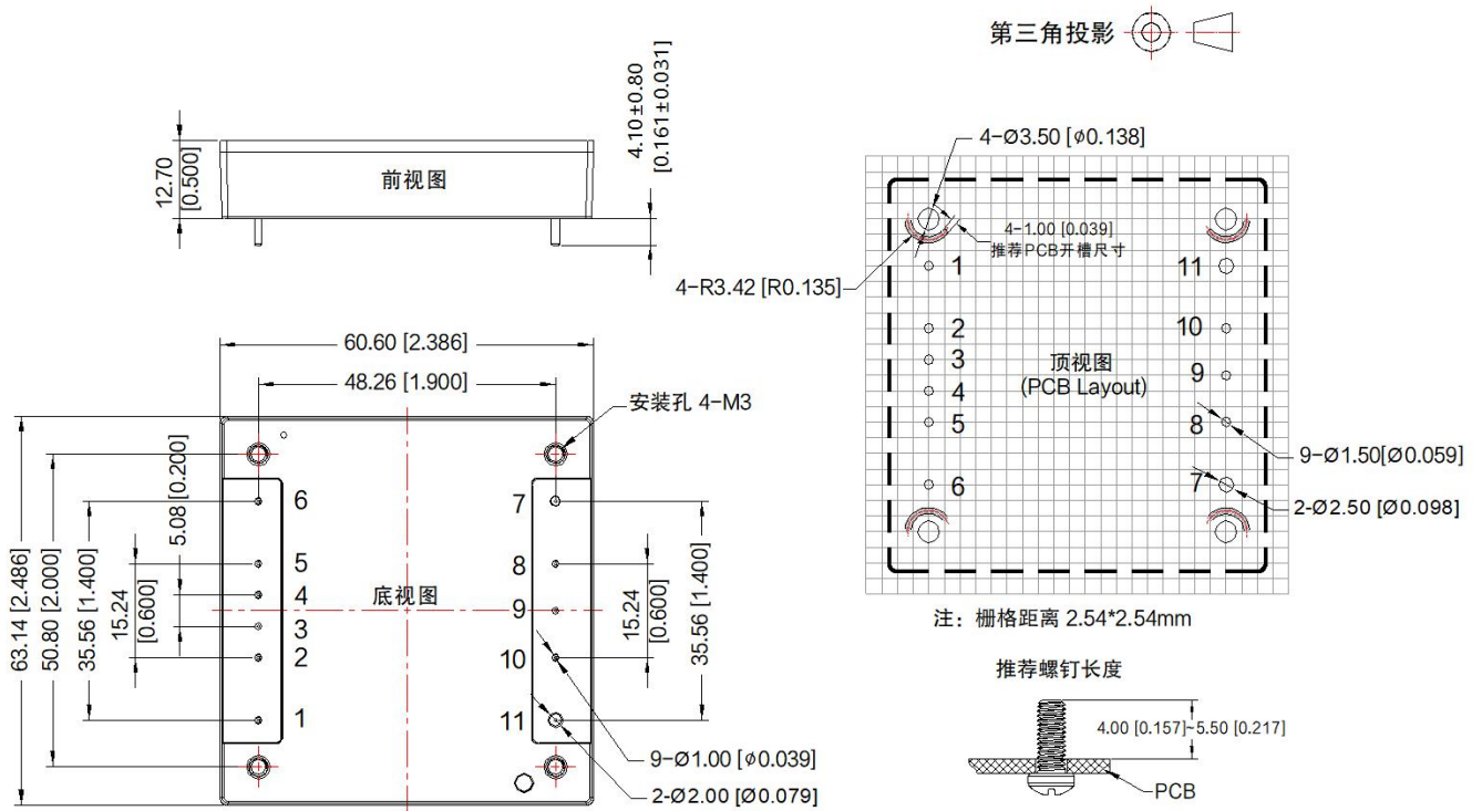
引脚方式
