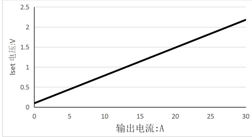
图 7 Iset 电压 Vs 输出电流
