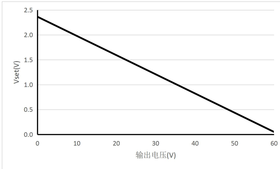
图 3 Vset 电压 Vs 输出电压
