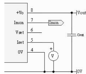
图 8 Iset 外部电源驱动接线图
