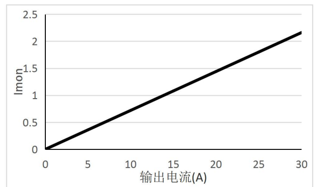
图 10 Imon Vs 输出电流
