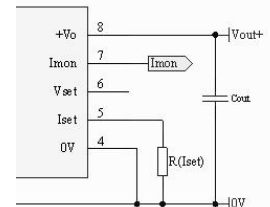
图 9 Iset 外接调整电阻接线图
