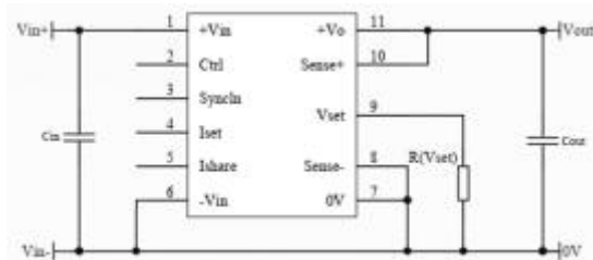
图5 Vset 外接调整电阻接线图
