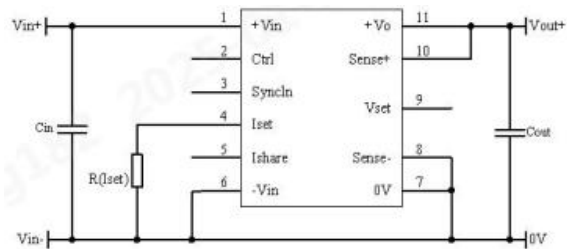
图 9 Iset 外接调整电阻接线图
