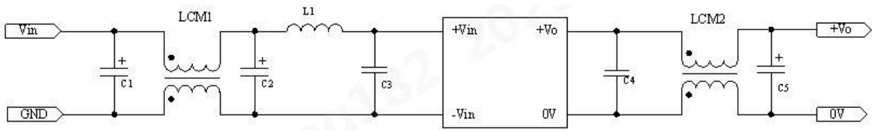
图 13 EMC 推荐电路
