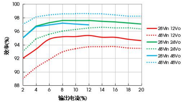
效率Vs输出负载
