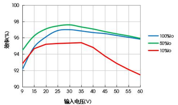
效率Vs输入电压 (Vo=24V)
