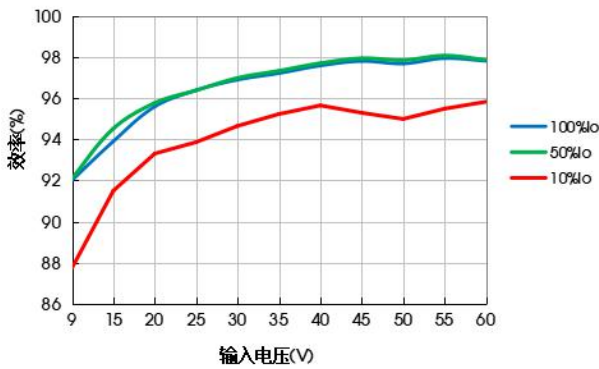
效率Vs输入电压 (Vo=48V)
