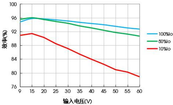
效率Vs输入电压 (Vo=12V)
