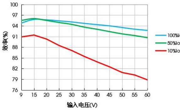
效率Vs输入电压 (Vo=12V)
