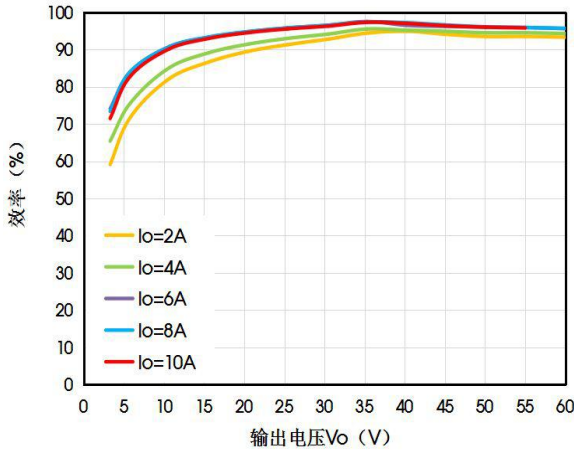
效率VS输出电压Vo (Vin=48V)
