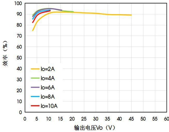
效率VS输出电压Vo (Vin=9V)
