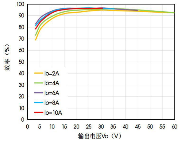
效率VS输出电压Vo (Vin=24V)
