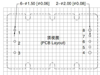
引脚方式
