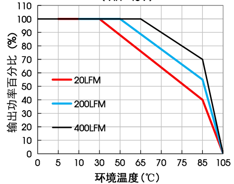
KJB4805EBF-20A 温度降额曲线 (Vin=48V)
