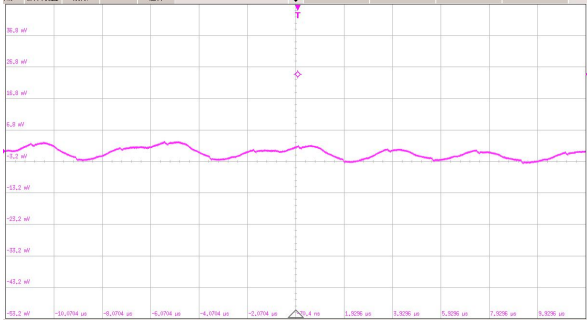
输出纹波&噪声 (10mV/div), 带宽: 20MHz
