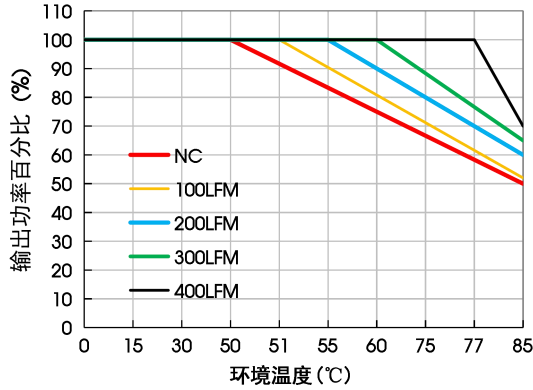
温度降额曲线 (Vo=1.0V)
