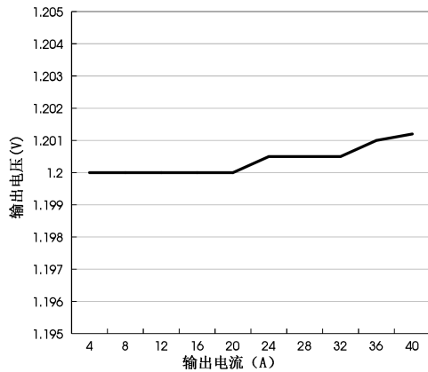
负载调节偏差
