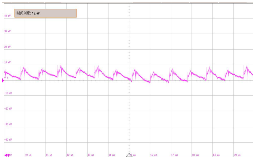
输出纹波&噪声 (10mV/div), 带宽: 20MHz
