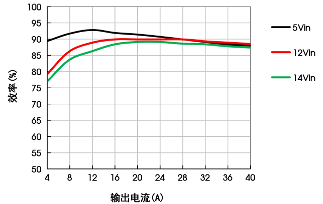
效率Vs输出负载 (Vout=1.0V)
