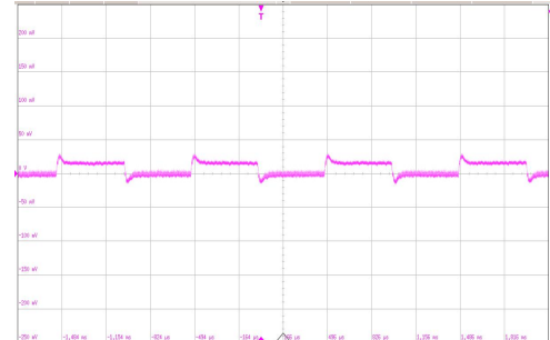
动态负载 (50mV/div), 2A/us, 10A-30A-10A 带宽: 20MHz
