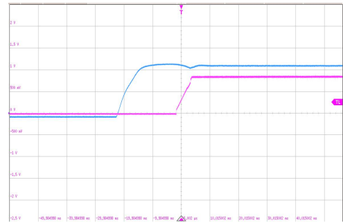
蓝: 输入电压, 红: 输出电压 (500mV/div), 时间 (10ms/div)
