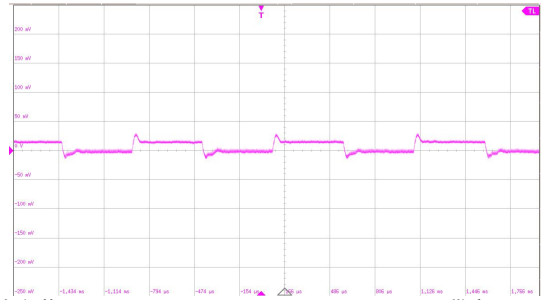
动态负载 (50mV/div), 2A/us, 10A-30A-10A, 带宽: 20MHz
