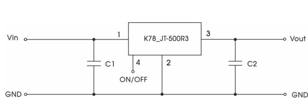
图 2 典型应用电路
