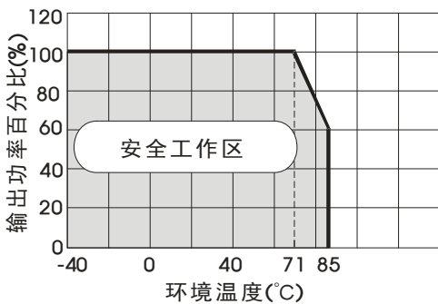
温度降额曲线
