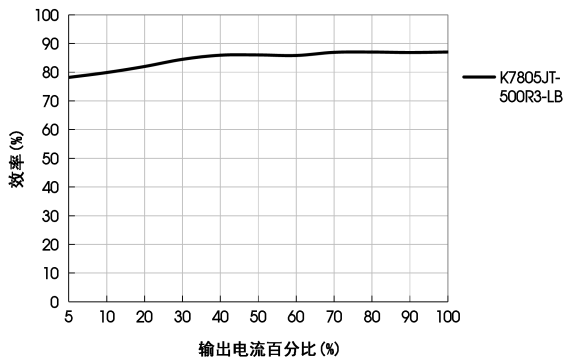
效率Vs输出负载 ( V_{in}=24\text{V} )
