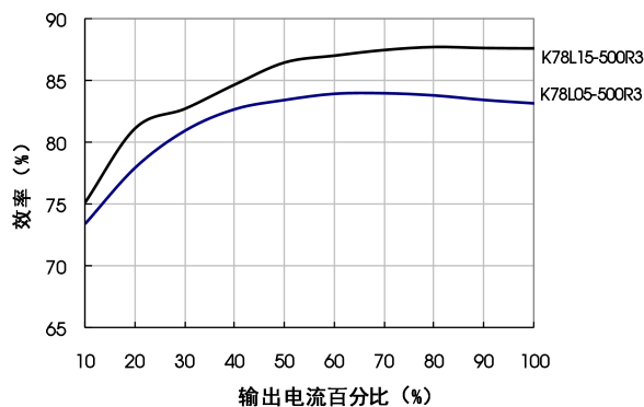
负输出效率Vs输出负载 (标称输入)
