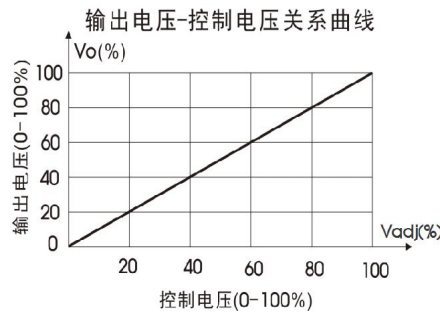
图 3 输出电压与控制电压关系曲线
