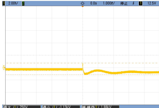
输出端电压波形(0.75KV)
