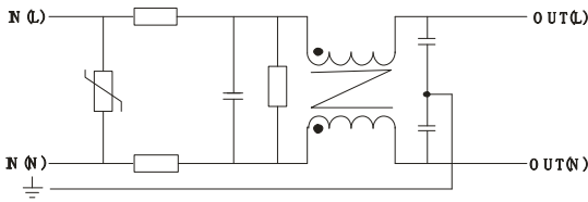
(图 1) FC-L01D
