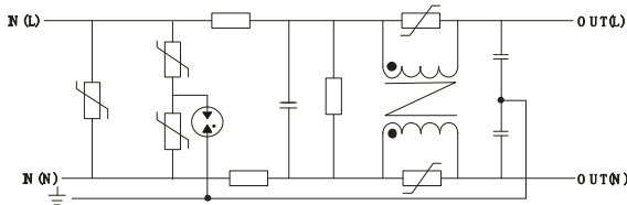
(图 2) FC-L01D2
