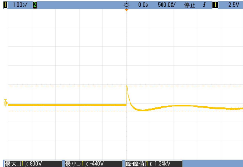
输出端电压波形(0.9KV)
