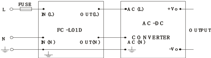
(图 1) FC-L01D
