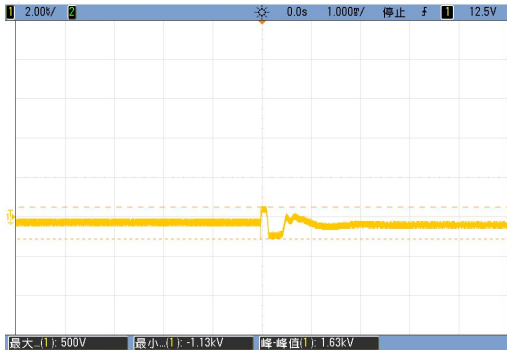
输出端电压波形(0.5KV)
