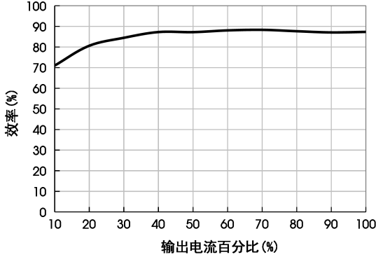
效率Vs输出负载 (Vin=5V)
